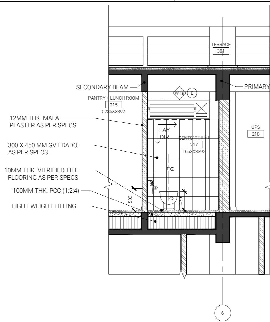
2 ELEVATION 1 1:50
