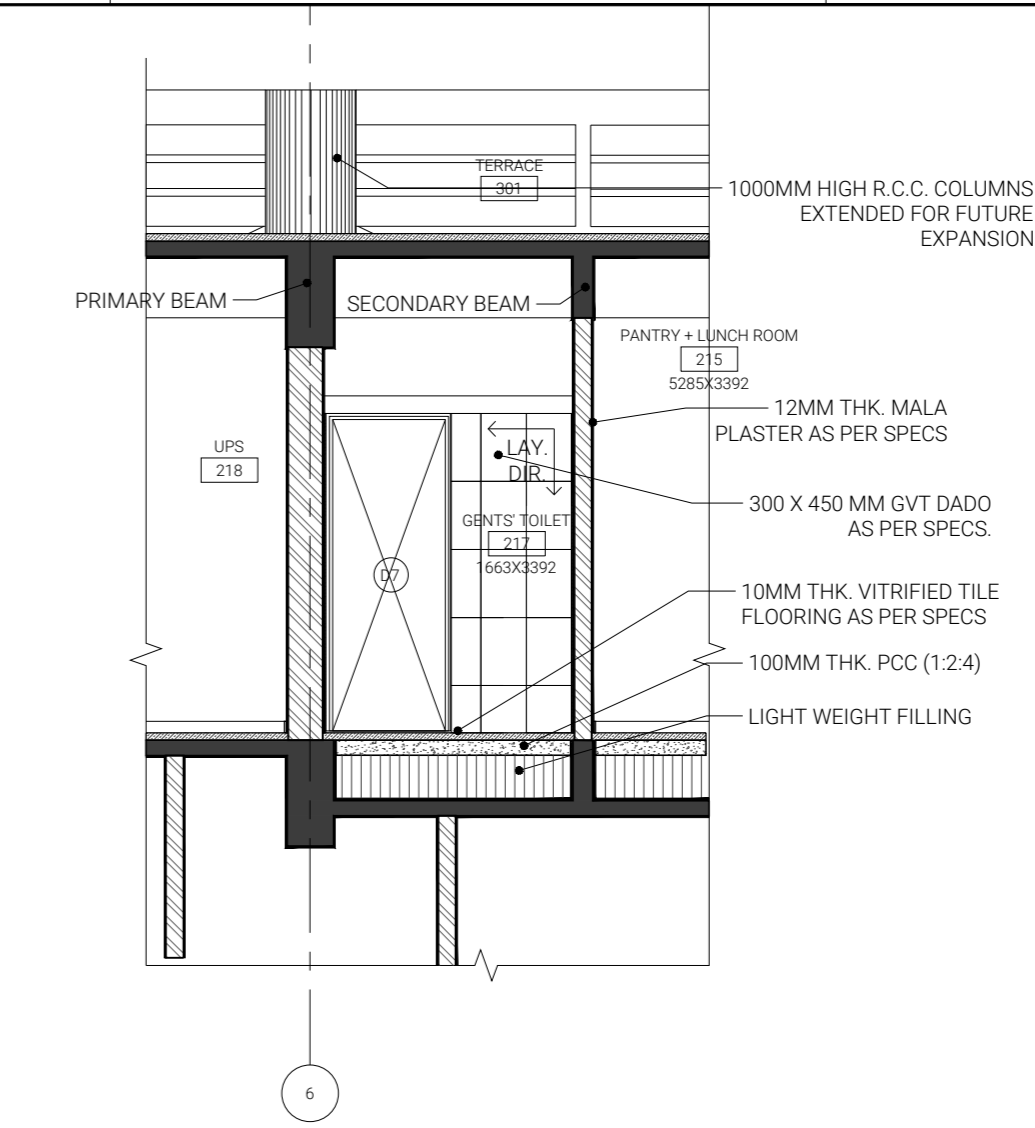
3 ELEVATION 3 1:50
