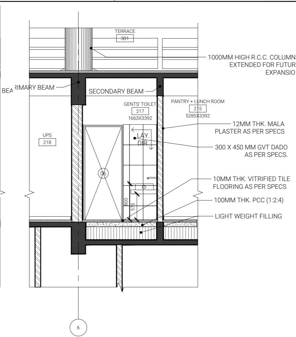
3 ELEVATION 3b 1:50
