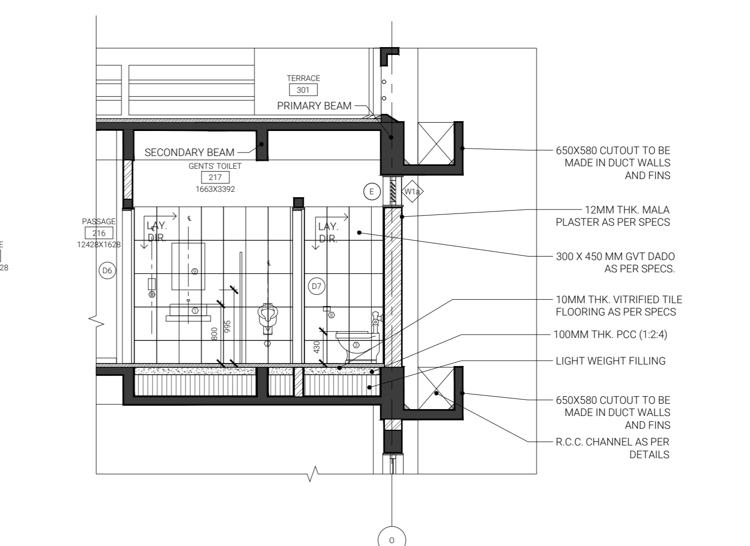
6 ELEVATION 2 1:50
